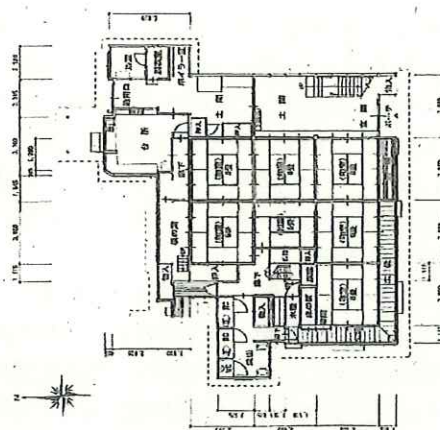
主屋1階平面図
