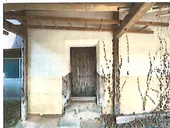
塩噌蔵・1階入り口構造
