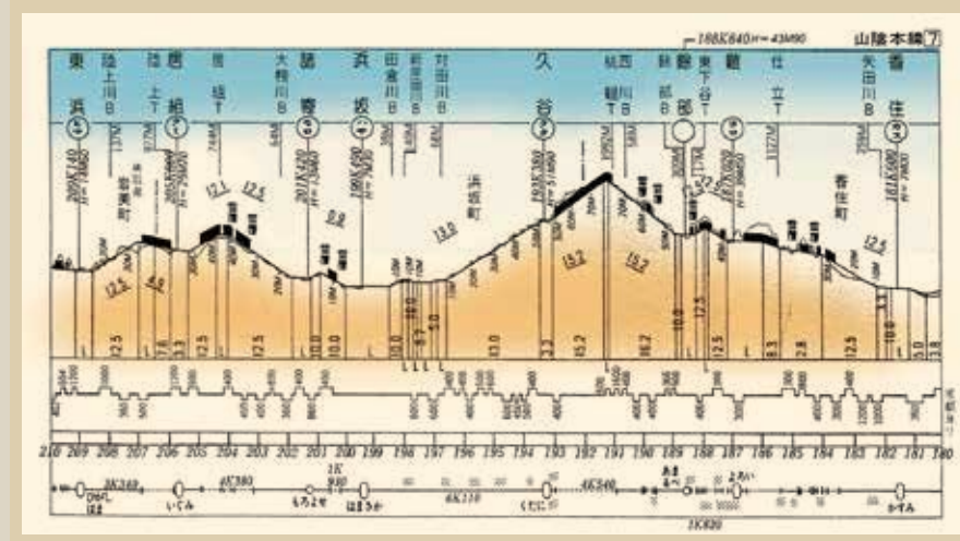
山陰線香住―浜坂間の線路縦断面図 (『日本鉄道名所一勾配・曲線の旅―7、山陽線・山陰線・予讃線』小学館、1994より)
