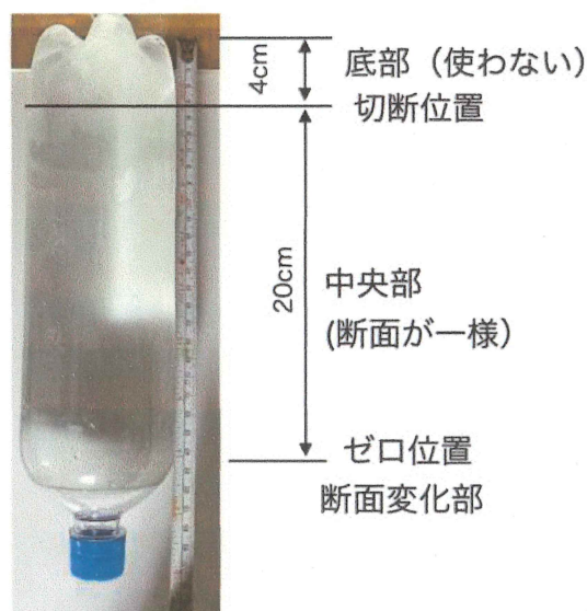
図2：上下逆さまに用いたペットボトル雨量計 (数値はペットボトルにより異なる)
