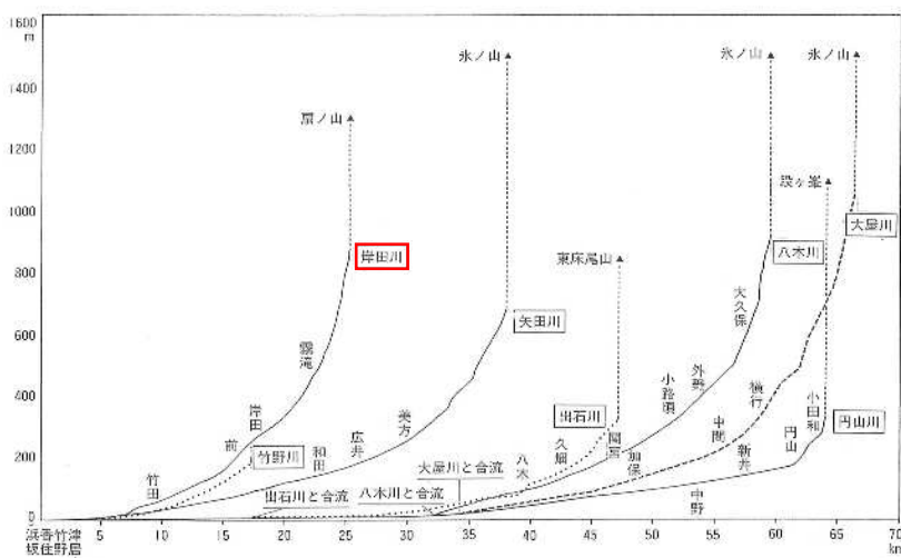
出典：『ひょうごの地形・地質・自然景観』田中真吾・中島和一編集、兵庫県監修 図6-1 但馬の河川の縦断面図
