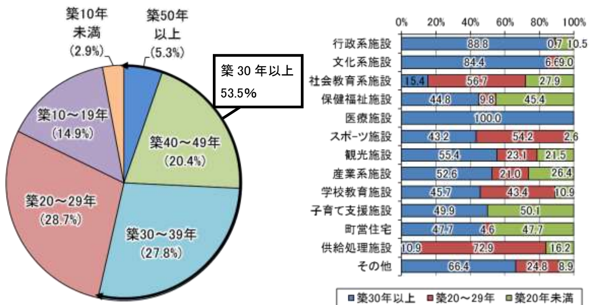
図表 2.7 建築年数別の延床面積
